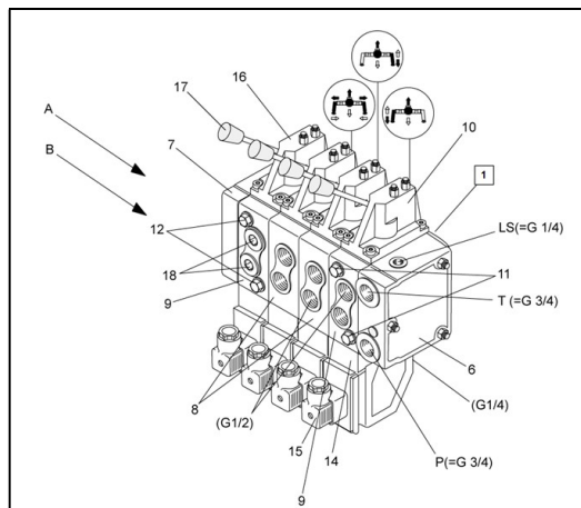
Общий вид распределителя PVG 32
