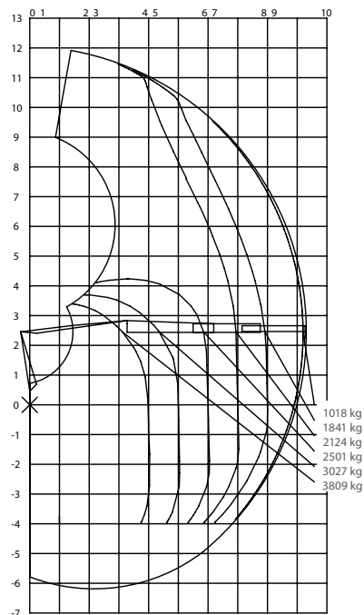
Load diagram F165Z93
