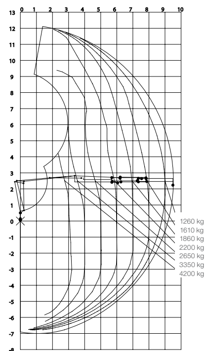
Load diagram J1500RZ 95
