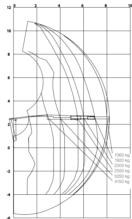
Load diagram J1500RZ 82
