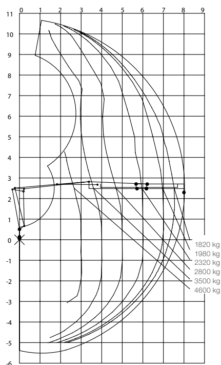
Load diagram J1500RZ 80
