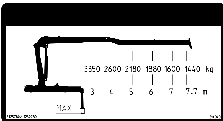
Load chart 1250Z80
