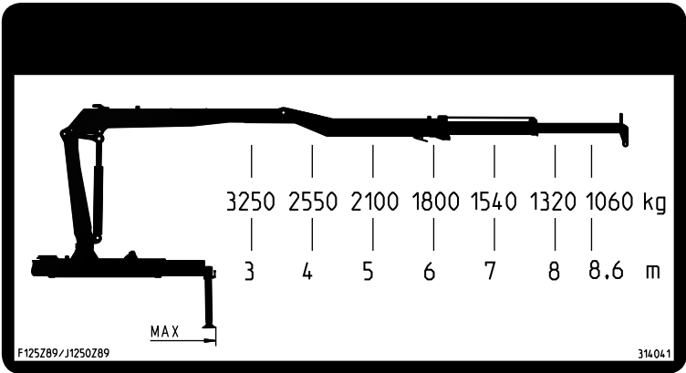
Load chart 1250Z89
