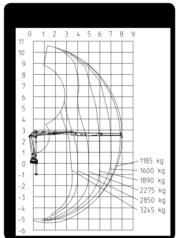
Load diagram 1250Z80
