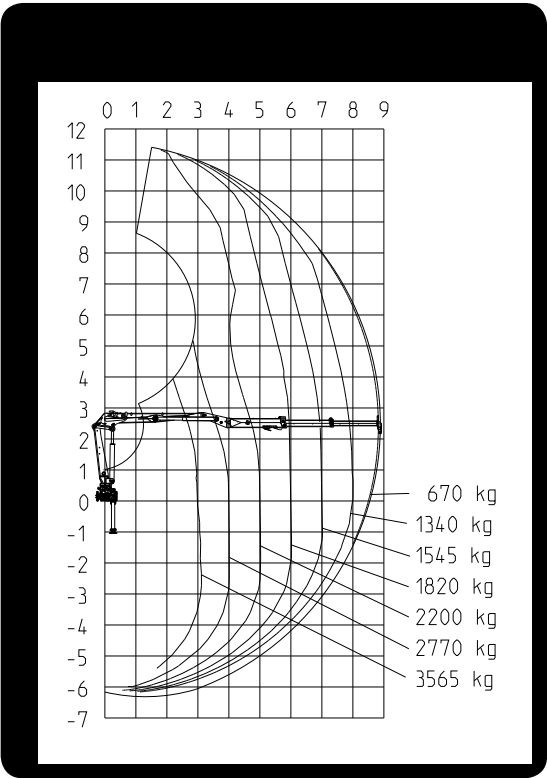
Load diagram 1250Z89
