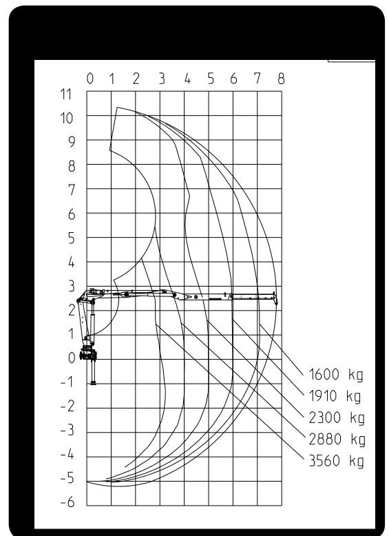
Load diagram 1250Z78
